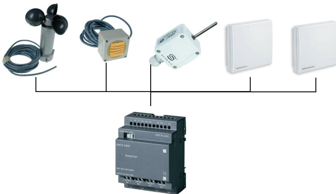
Logique de gestion FREECOOLING
